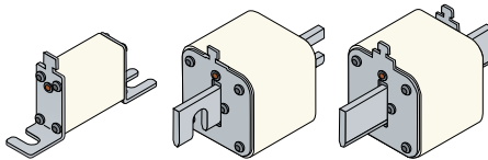
Fyrkantsäkringar slitsad L-kontaktskena DIN 43653
